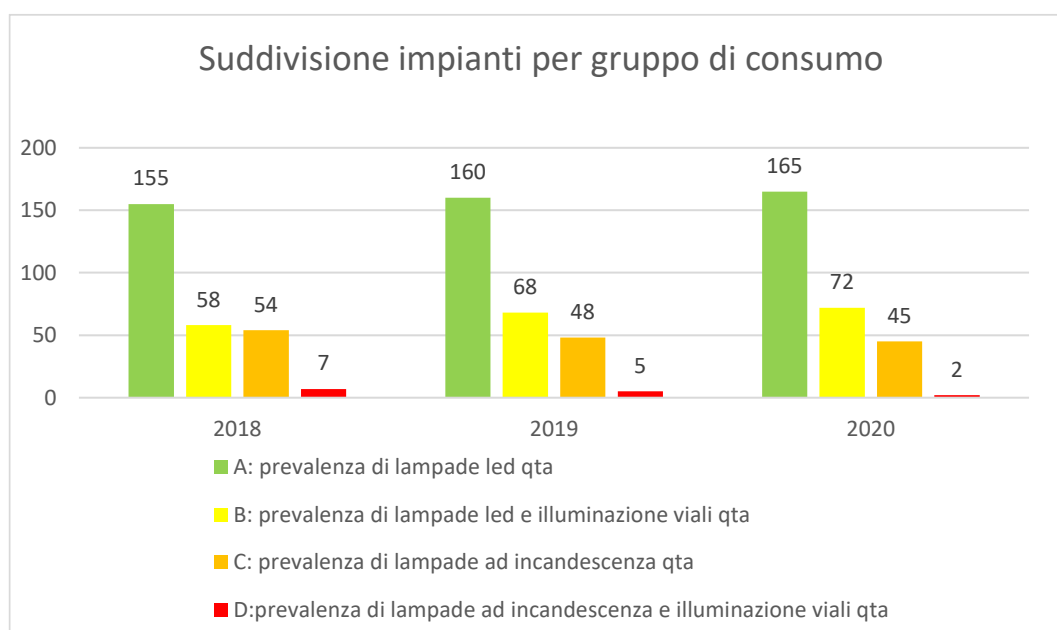
Figura 4: suddivisione impianti per gruppo di consumo (kWh/numero punti luce) ovvero prevalenza di tecnologia
